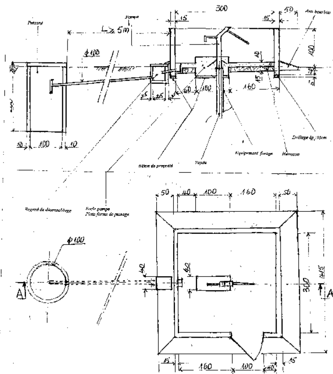
STRUCTURE DE SURFACE D'UN FORAGE
